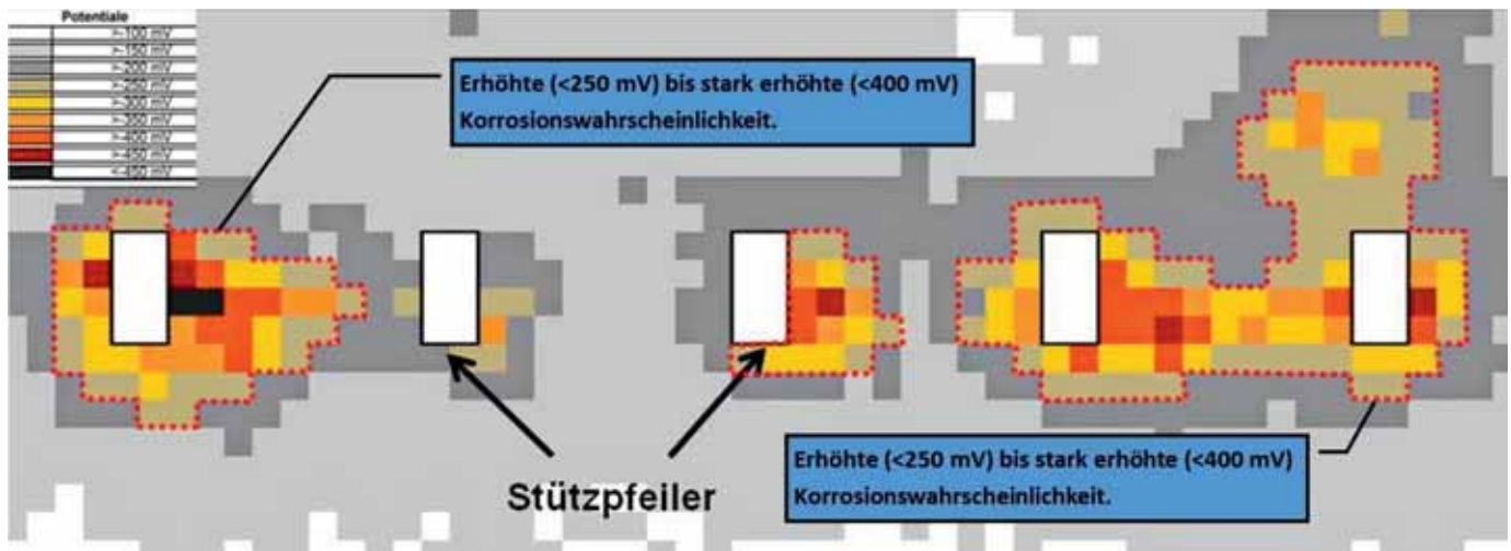
Abb. 1 Die Darstellung zeigt das Ergebnis der sogenannten elektrischen Potentialfeldmessung in einer der Tiefgaragen vor der Instandsetzung. Bei diesem Verfahren wurden die Bodenflächen mit einer
